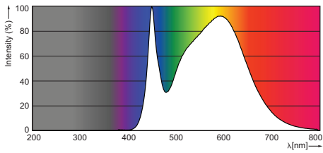
LEDtube 900mm 15W /840 T8C Rot
